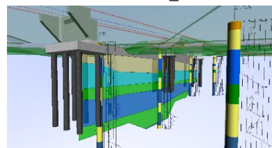
3D地層モデリング GEO_Kit
