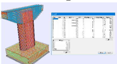
3D配筋モデリング RC_Kit
