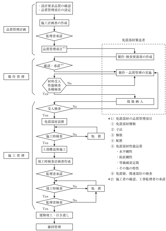
図 2.1.2 免震建築物の品質管理フロー
